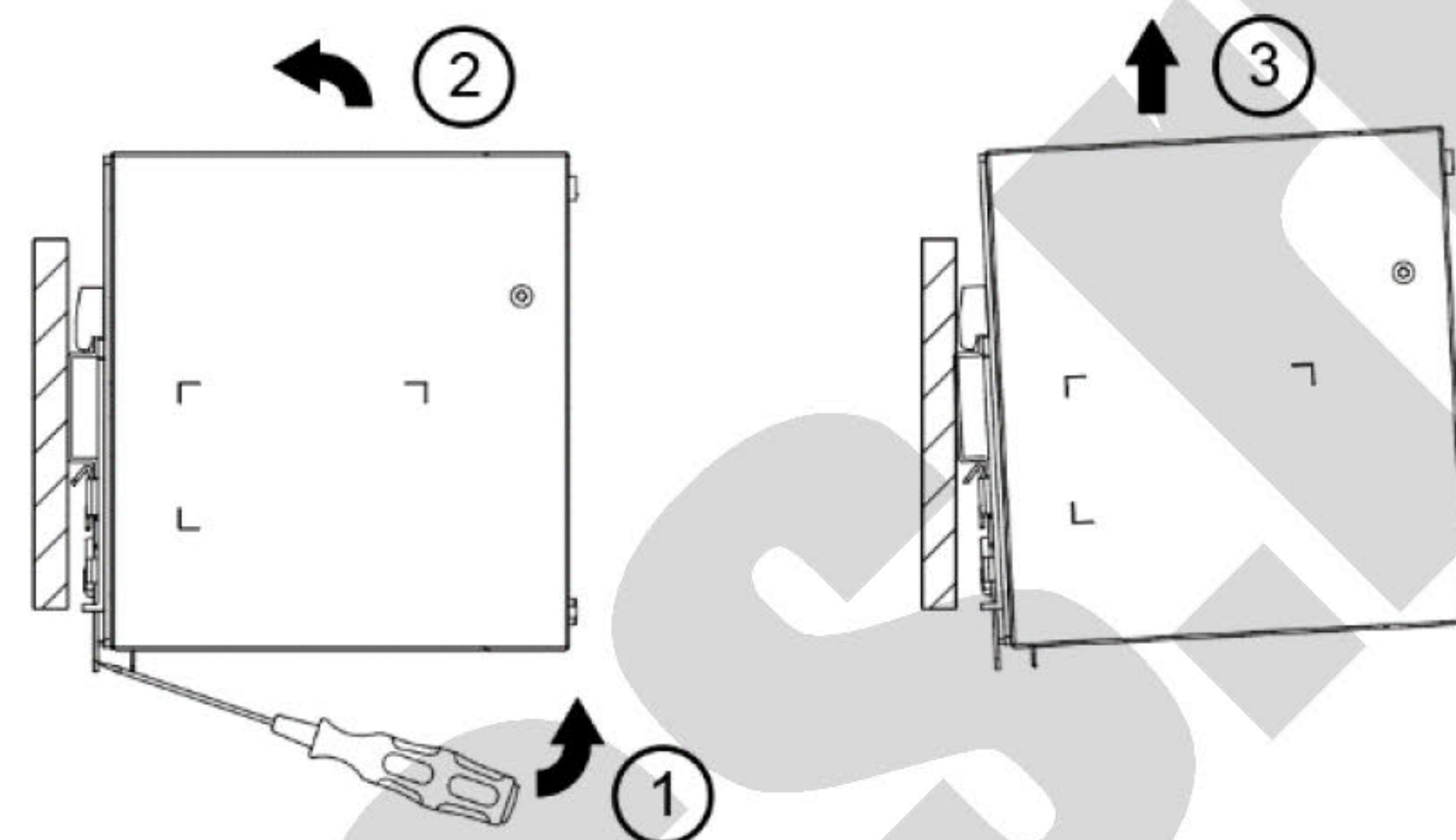
Рис. 3.2 Демонтаж
