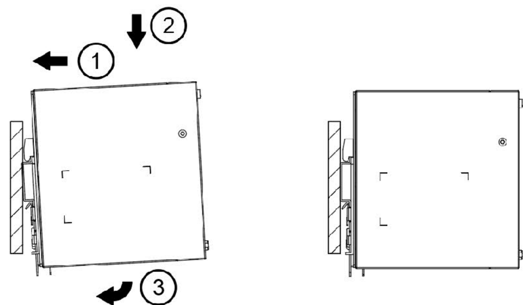
Рис. 3.1 Монтаж
